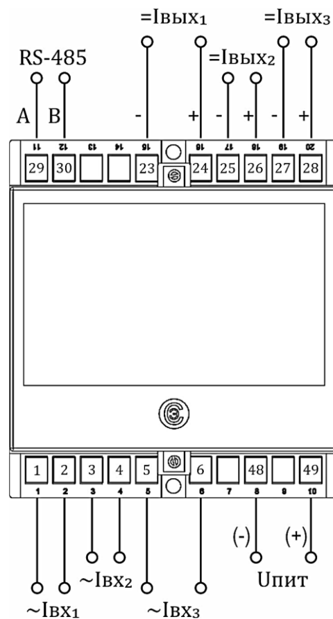
б) Корпус EB20 (3 входа, 3 аналоговых выхода, 1 порт RS-485)
