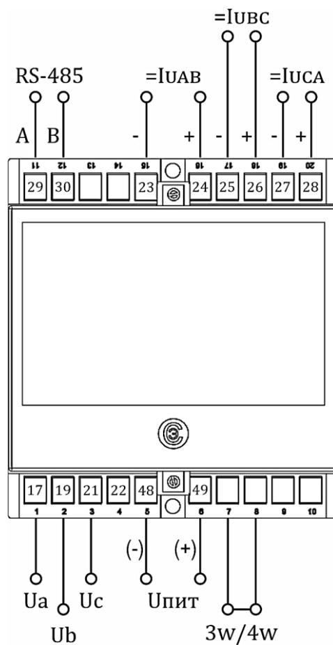
б) Корпус EB20
