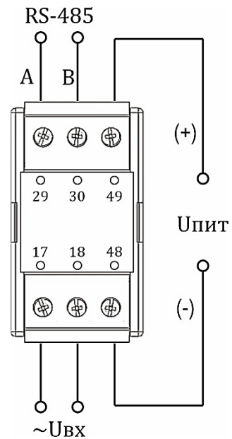
б) Корпус М6 (1 вход, 1 порт RS-485)
