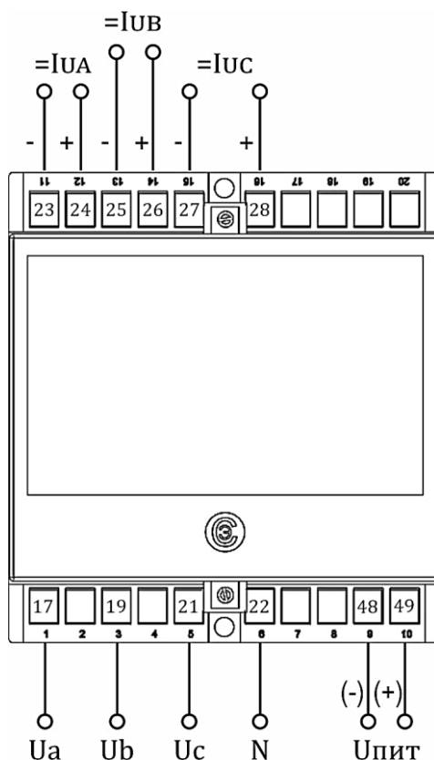
Копус E20 (3 входа с объединенной нейтралью, 3 аналоговых выхода)
