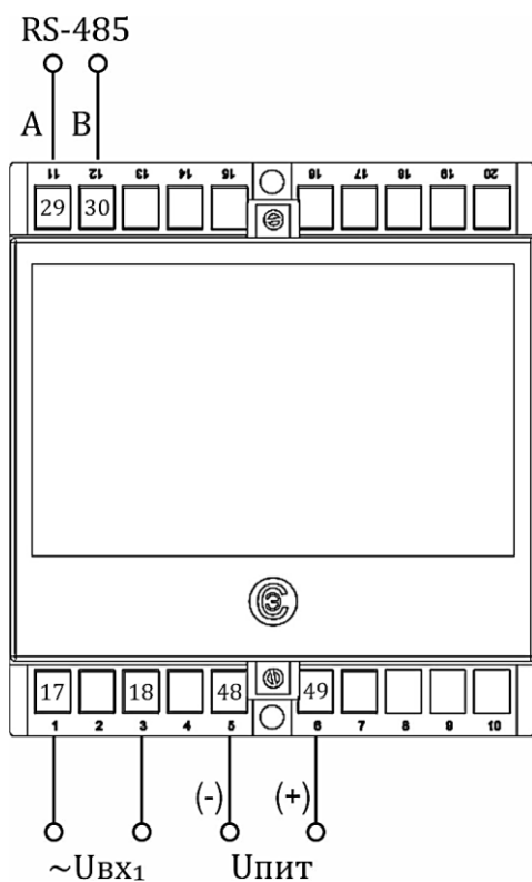
а) Корпус E20 (1 вход, 1 порт RS-485)
