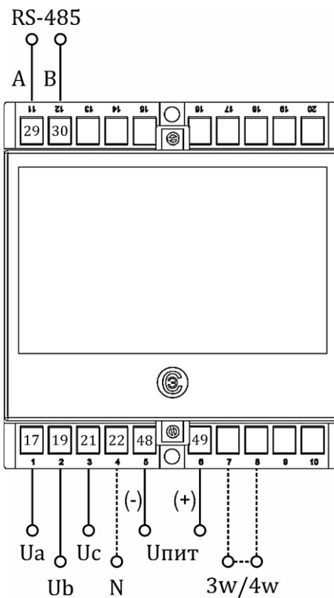
Корпус EB20 (3 входа с объединенной нейтралью, 1 порт RS-485 )
