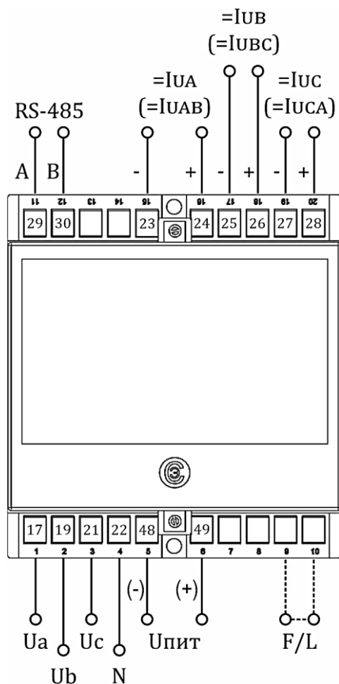
а) Корпус EB20
