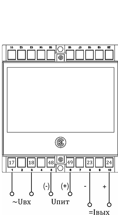
а) Корпус Е20 (1 вход, 1 аналоговый выход)
