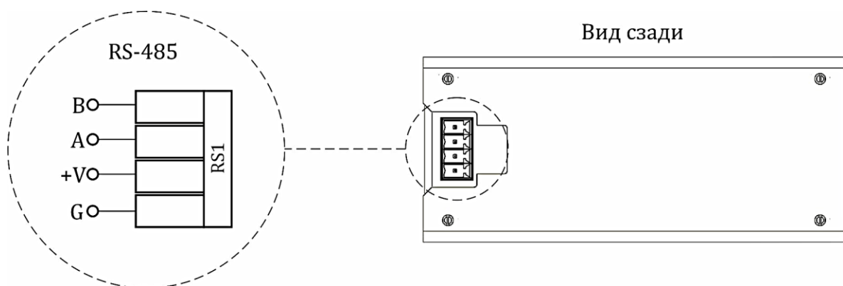
Рисунок Б.9 – Схемы электрические подключения E8DU
